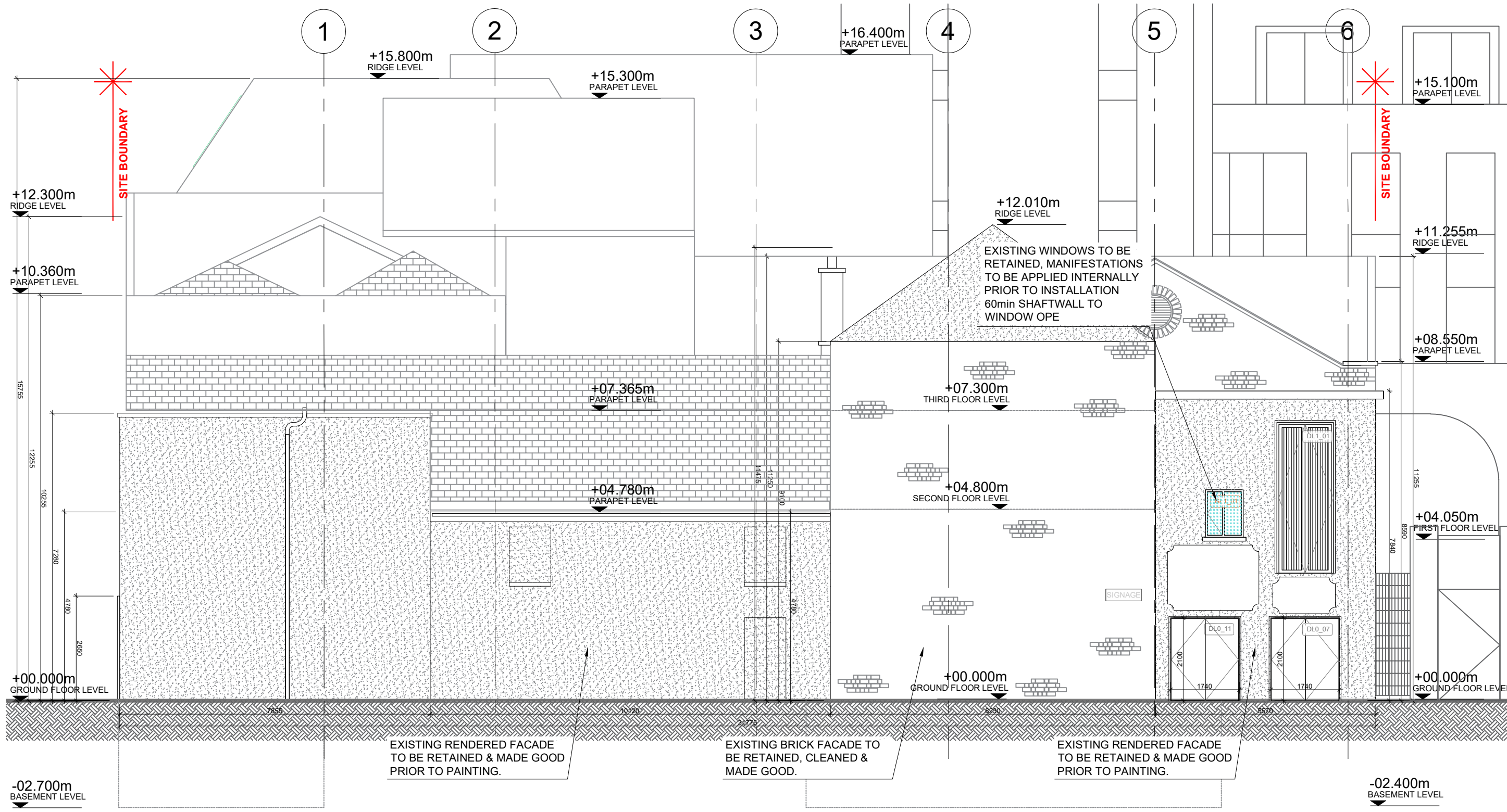
3 30.10 WEST ELEVATION_TALBOT LANE SCALE: 1:100
